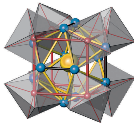
Blick in ein Skutterudit mit Füllung: Die roten Kugeln stehen für Kobalt-, Rhodium- oder Iridiumatome, die blauen für Phosphor, Arsen oder Antimon. In den Hohlräumen des Gerüsts finden Calcium- oder Bariumatome (gelb) Platz. In Grau sind oktaedrische Strukturelemente angedeutet.
